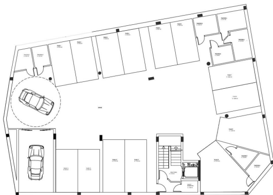
PLANTA SOTANO
