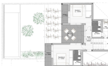
PLANTA PRIMERA
