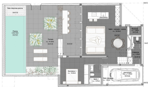
PLANTA BAJA
