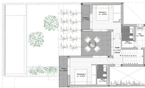
PLANTA PRIMERA
